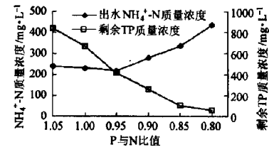
图13 不同P与N比值下鸟粪石处理效果曲线
