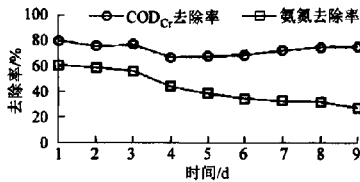
图10 工艺2 SBR运行效果曲线
