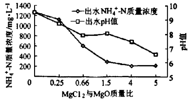
图11 不同 MgCl_2 与 MgO 比值时鸟粪石处理效果曲线
