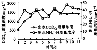
图 14 工艺 3 的 SBR 处理效果曲线 Fig. 14 Effect of SBR at stage three
