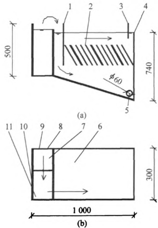
图 3 混凝装置示意图
