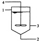
图 1 鸟粪石反应器示意图
