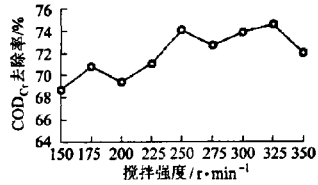
图6 不同搅拌强度的混凝效果曲线 Fig. 6 Coagulation effect in different stirring intensities
