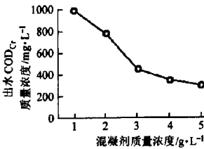
图 15 SBR 出水不同混凝剂质量浓度处理效果曲线 Fig. 15 Effect of SBR effluent coagulation in different coagulant concentrations
