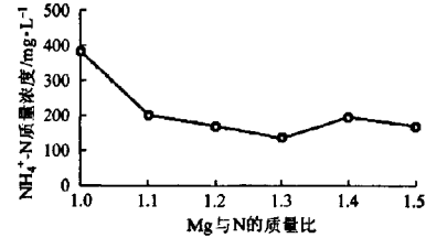
图12 不同Mg与N比值下鸟粪石处理效果曲线
