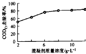
图4 不同混凝剂质量浓度的混凝效果曲线 Fig. 4 Coagulation effect in different coagulant concentrations
