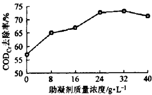
图5 不同助凝剂质量浓度的混凝效果曲线 Fig. 5 Coagulation effect in different coagulant aid concentrations
