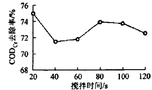
图7 不同搅拌时间的混凝效果曲线 Fig. 7 Coagulation effect at different stirring time
