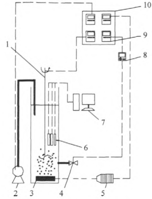
图 2 SBR 反应器示意图
